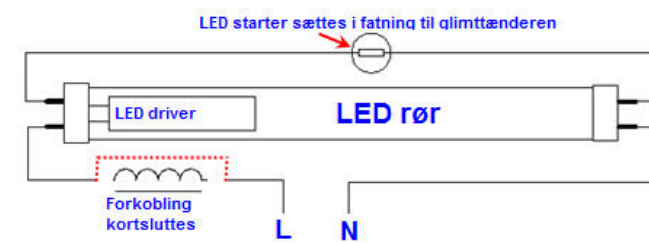
Diagram for kortslutning af magnetisk forkobling med spole og kondensator i et T8 armatur.
