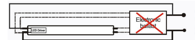
Diagram for kortslutning af HF forkobling i T8 armatur. Her skal kabelføringen ændres, så single-end LED røret kun får stel og fase i den ene ende. Husk at vende røret rigtigt, da der ellers sker kortslutning.
